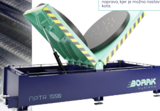
Prekucnik Patentirana naprava za prevračanje, obračanje in obdelavo težkih elementov. Omogoča 360° obračanje po X in Y osi, obenem lahko služi kot dvojno delovno mesto. Možna je manipulacija najrazličnejših oblik, velikosti in bremen - od 100 kg - 10 t serijsko, ostalo po naročilu. Deluje v manj zahtevnih kot zelo zahtevnih delovnih okoljih, na delovnih mestih kot so varjenje, sestava ali popravilo orodij ... Lahko deluje tudi kot CNC naprava, kjer je možna nastavitve poljubnega kota.
