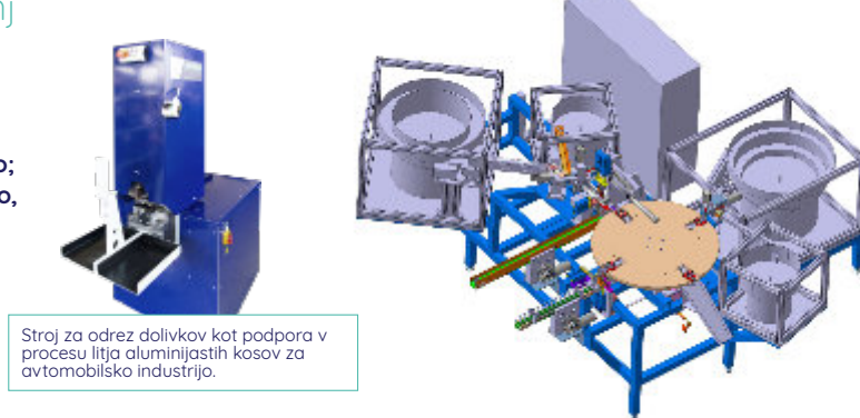
Avtomatski stroj za sestavo nosilca radiatorja iz šestih sestavnih delov.
